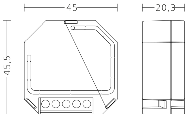
Dibujo acotado
