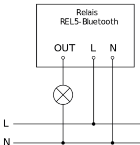
Diagrama electrónico 1
